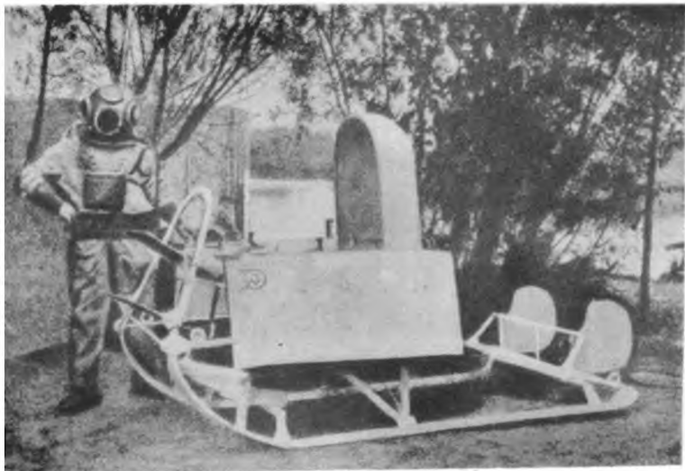
Водолазные санки (видъ сбоку).
