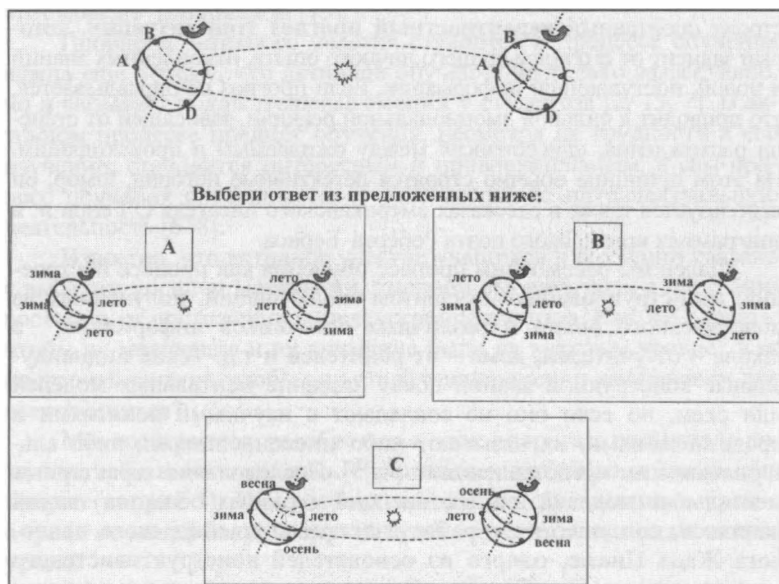
Рис. 1. Здесь изображены два положения земного шара на орбите вокруг Солнца. Какие времена года в отмеченных точках?
