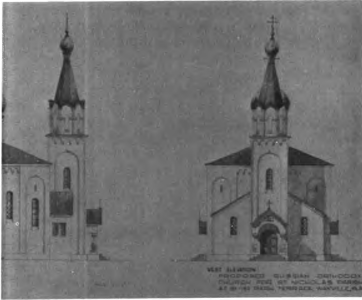
Проектъ новаго храма.
