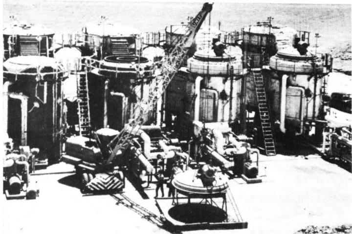
Экспериментальная опреснительная установка (по методу А.Зархина) в Эйлате.
